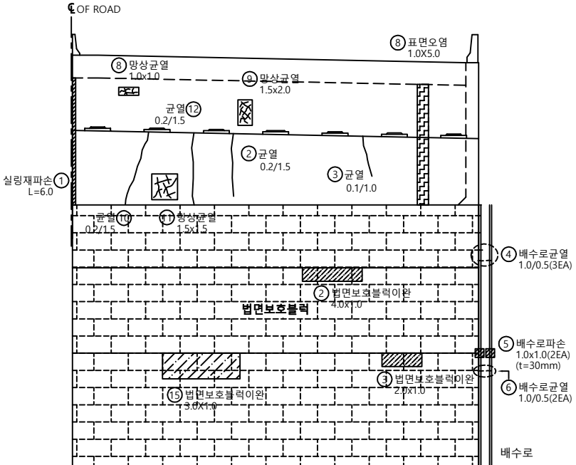
정면도
